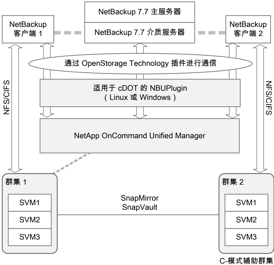
图 11-2 NetBackup 与适用于 Clustered Data ONTAP 的 NBUPlugin 之间的通信
