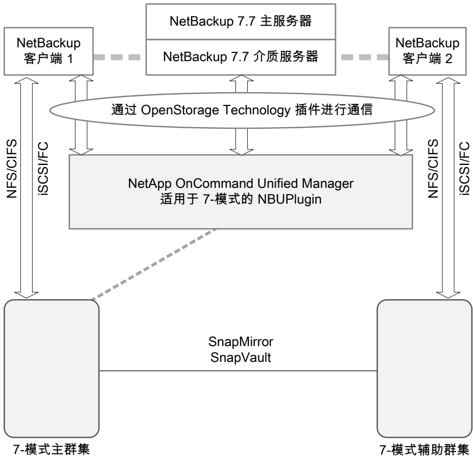
图 11-1 NetBackup 与适用于 7-Mode 的 NBUPlugin 之间的通信
