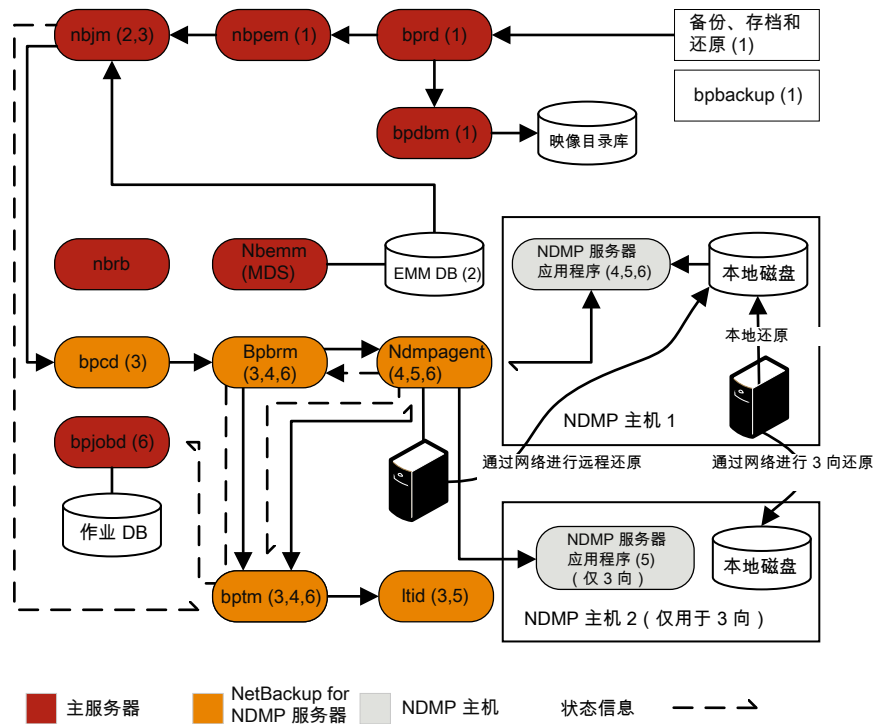
图 6-2 NDMP 还原进程
