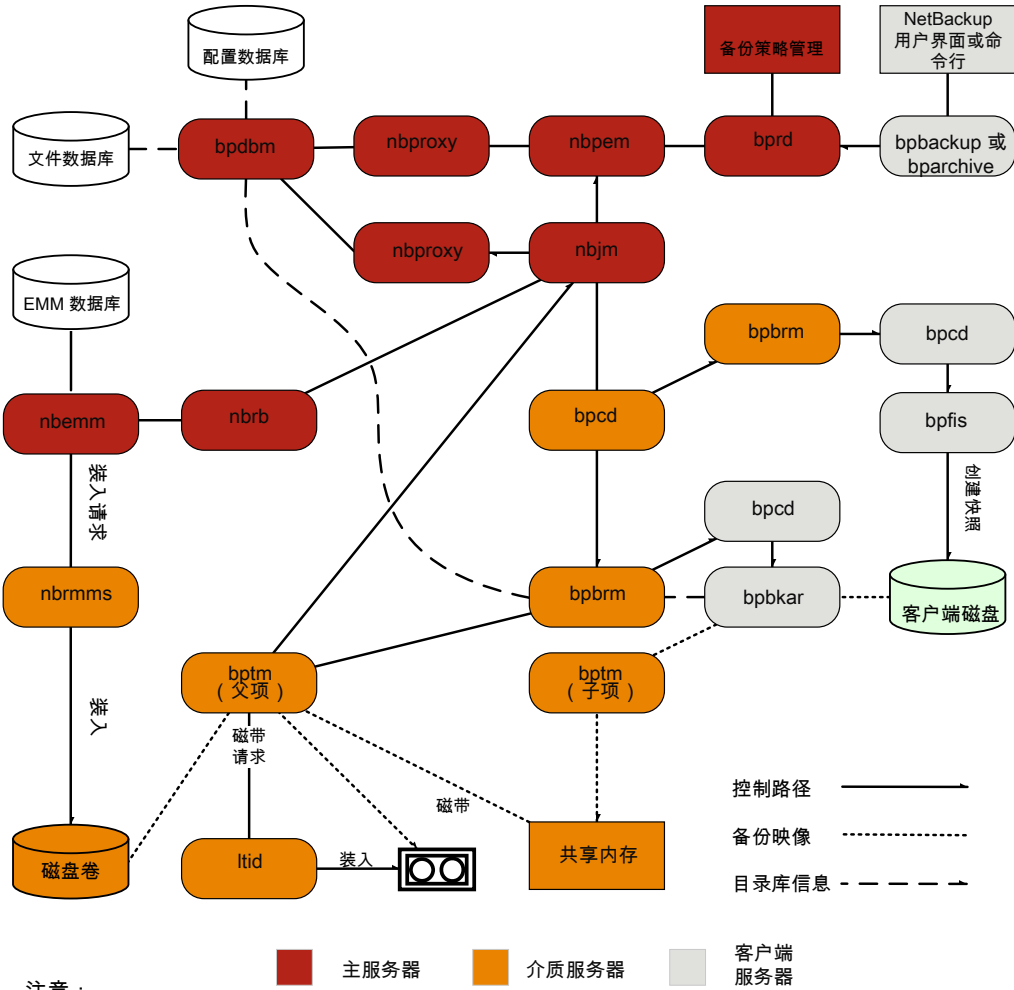
图 9-1 快照备份和使用多个数据流的 Windows Open File Backup
