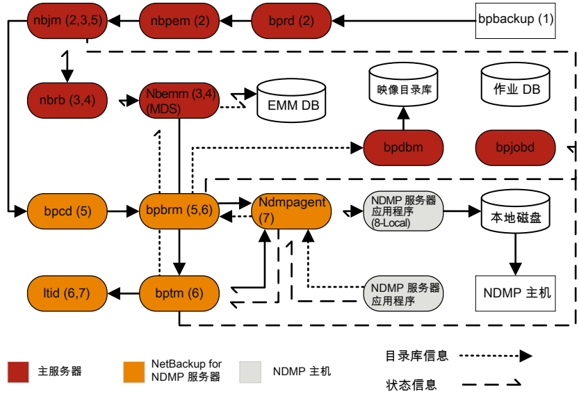
图 6-1 NDMP 备份进程
