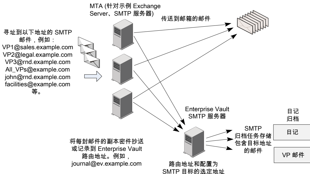
图 2-3 SMTP 组日记记录示例
