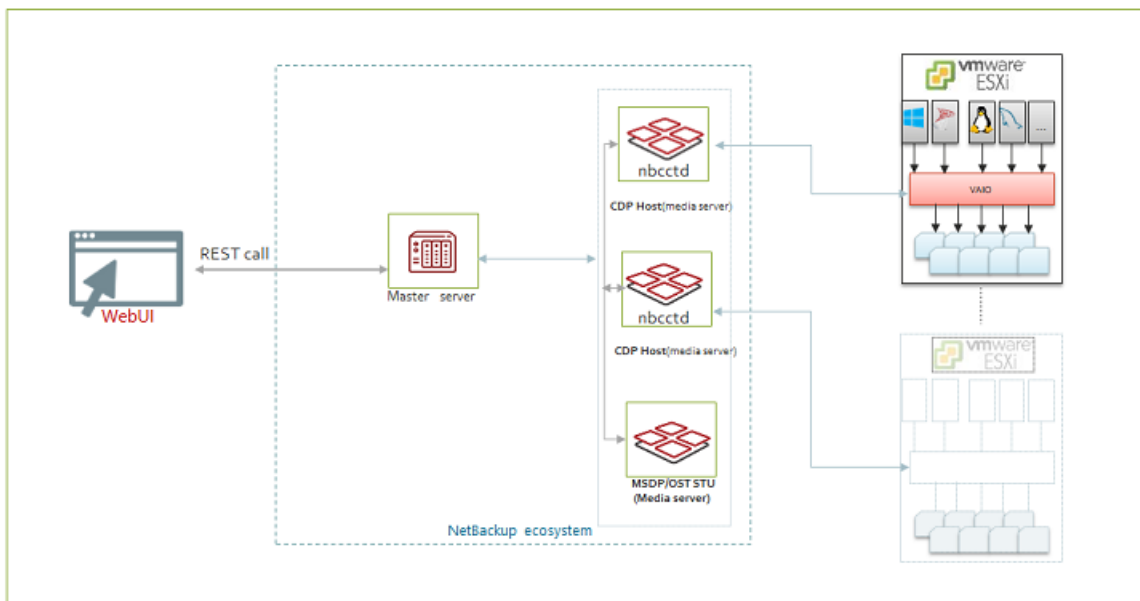
图 7-1 CDP 体系结构
