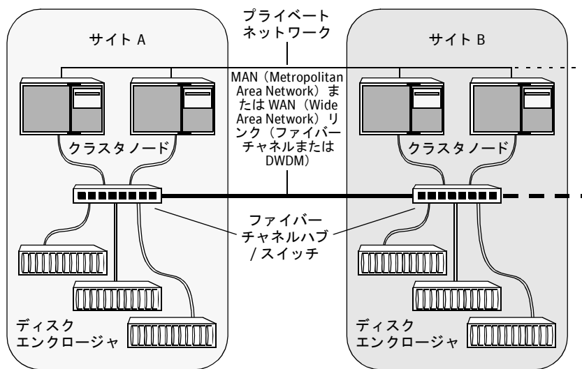
図 5-1 2 サイトのリモートミラー設定の例
