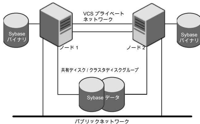
図 1-2 ローカルディスク上のバイナリおよび共用ディスク上の Sybase データ
