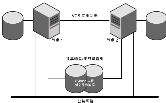
图 1-1 Sybase 二进制文件和数据位于共享磁盘上
