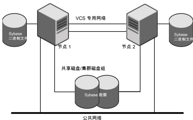
图 1-2 二进制文件位于本地磁盘上，而 Sybase 数据位于共享磁盘上
