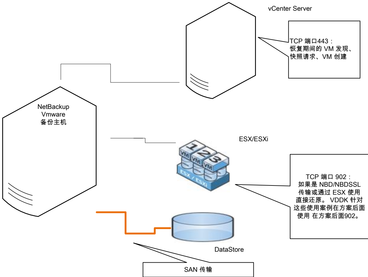
使用物理 VMware 备份主机的 SAN 和 NBD 传输
