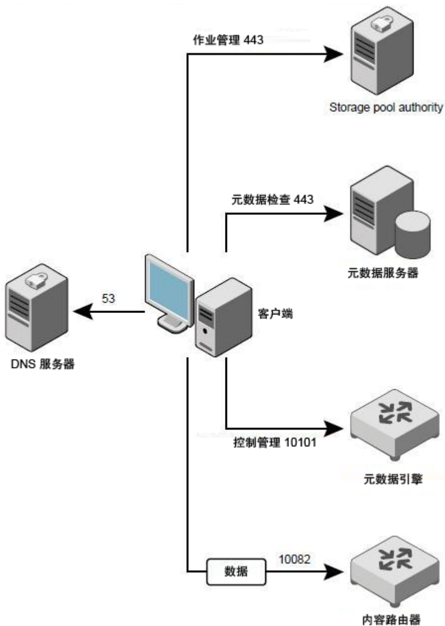
图 3-2 通信端口
